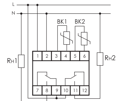
Схема подключения при нагрузке до 16А.
