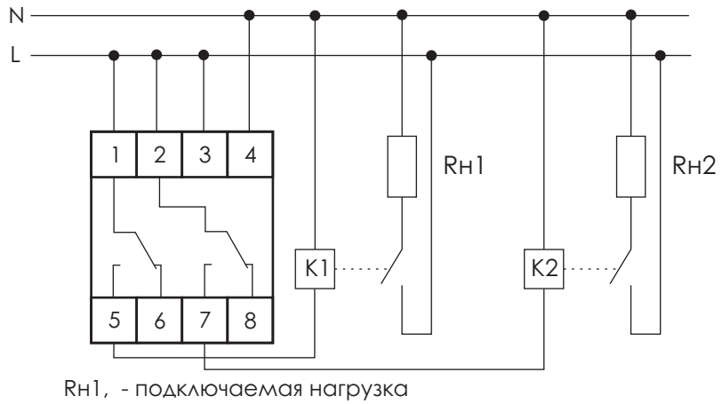
Рис.4 Схема подключения изделия с использованием контактора ток нагрузки более 16А.
